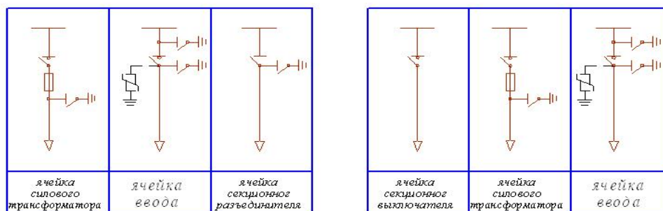
УВН по тупиковой схеме
