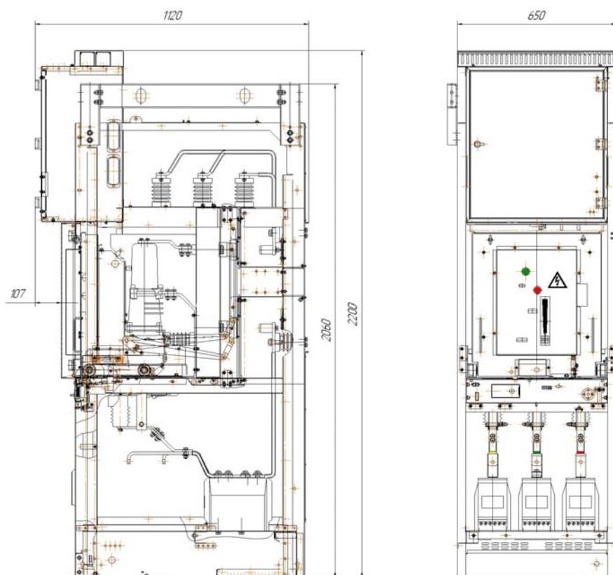
Рисунок 6.1 – Общий вид КСО-СЭЩ®-298 MSC
